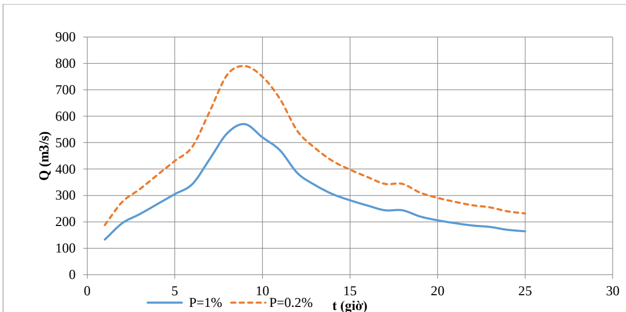
Phụ lục 5 : Biểu đồ tần suất lũ công trình thủy điện Nậm Chim 1A
